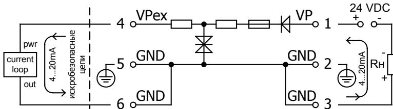
Барьер искрозащиты BSZ.621.105.242
