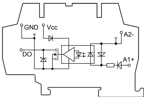
Рис. 4.1 Функциональная схема модуля гальванической развязки
