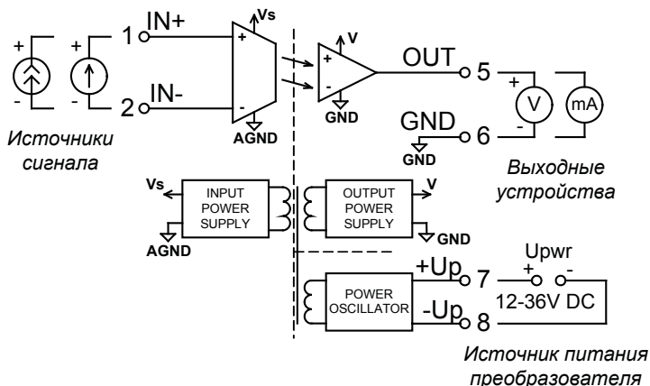
Рис. 4.1 Преобразователь сигналов CSG.125. Структурная схема и схема подключения
