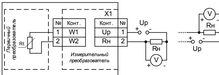
Рис. 4.1 Схема подключения термопреобразователя
